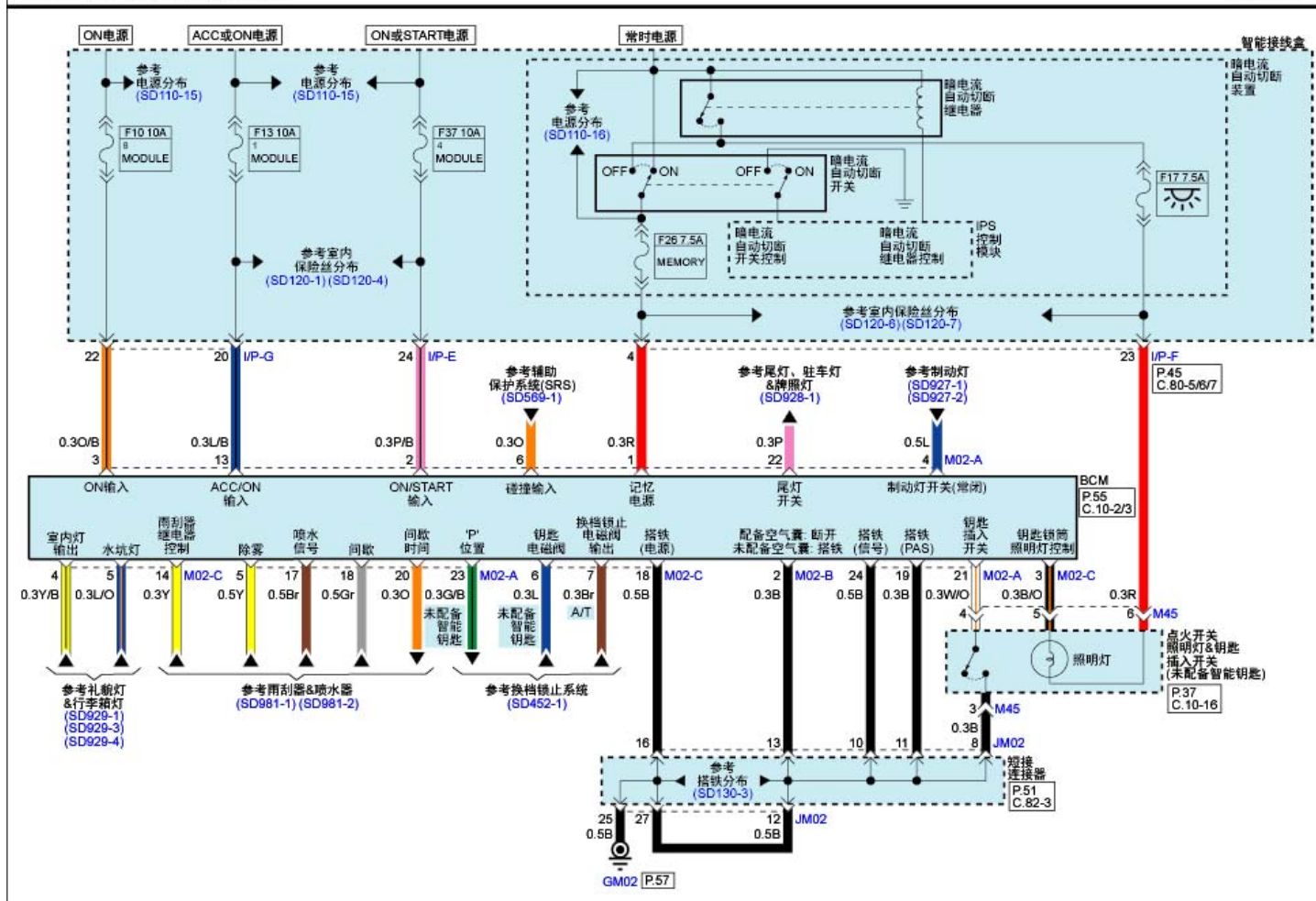
车身控制模块(BCM)系统(1)
